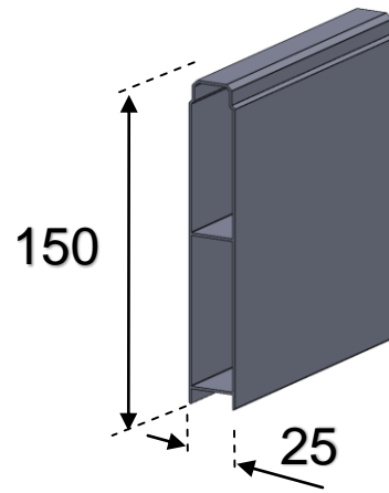
Lame pleine 150mm ép. 25mm
