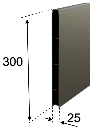
Lame pleine 300mm ép. 25mm
